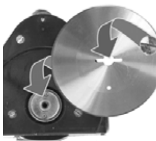
Das neue Schneidmesser anlegen bzw. die Haltescheibe und die Befestigungsschraube anschrauben.
